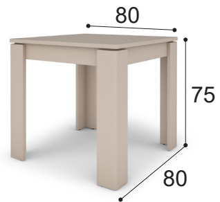
Avola TB 80x80
