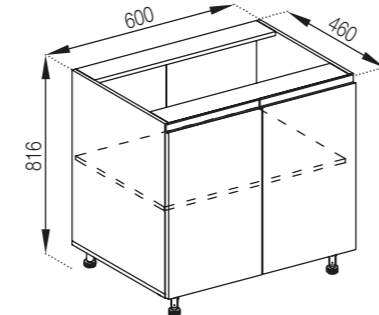
D 60
