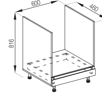
D 60 R
